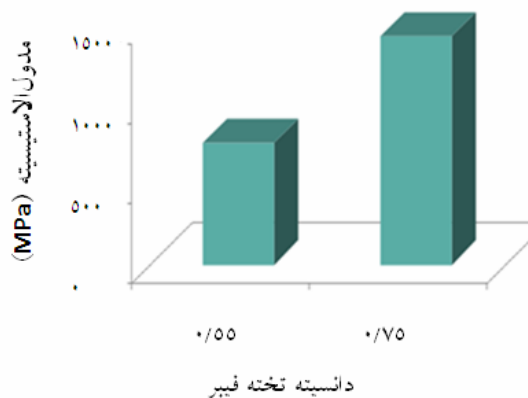
شکل ۳- اثر مستقل دانسیته و نوع فیبر بر مدول الاستیسیتة تخته فیبرهای آزمونی
