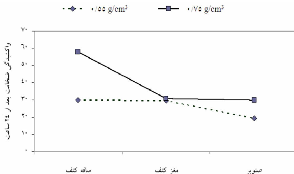
شکل ۶- اثر متقابل دانسیته تخته و نوع الیاف لیگنوسلولزی بر واکشیدگی ضخامت بعد از ۲۴ ساعت غوطه‌وری در آب تخته‌فیبرهای آزمونی
