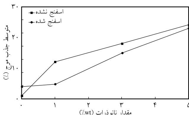
شکل ۴- متوسط مقدار جذب موج تابشی در نمونه‌ها در بازه بسامد ۸-۱۲ GHz
