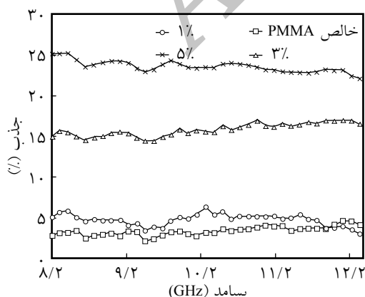
شکل ۶- مقدار جذب اسفنج‌های پلی‌متیل متاکریلات خالص و حاوی مقادیر مختلف نانوذرات در بازه بسامد ۸-۱۲ GHz
