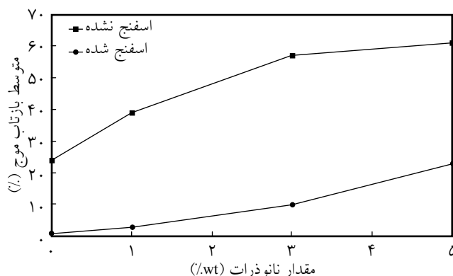
شکل ۳- متوسط مقدار بازتاب موج تابشی به نمونه‌ها در بازه بسامد ۸-۱۲ GHz
