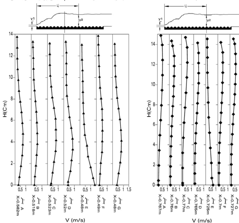
ادامه شکل ۱۰- پروفیل‌های سرعت روی بستر افقی موج‌دار در سه مقطع، یک سوم ابتدای پرش، یک سوم میانی و یک سوم انتهایی پرش روی بسترهای موج‌دار سینوسی
