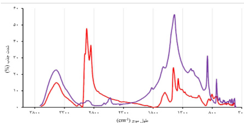
شکل ۱۶ طیف‌سنجی فرورسرخ (FTIR) نمونه مغزه اشباع از نفت خام (قرمز) و نمونه مغزه بعد از تزریق فیلترات سیال حفاری (آبی)
