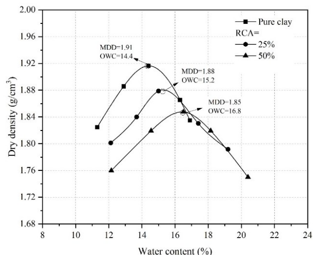
شکل ۳. منحنی تراکم مخلوط رس و RCA
