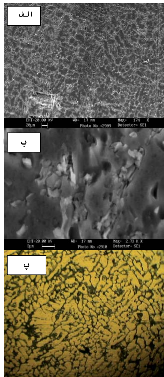
شکل (۵): ریزساختار نمونه‌های ریخته‌گری شده در دمای 850^{\circ}\text{C} با اندازه ذرات 300\mu\text{m} : (الف) تصویر SEM با بزرگنمایی 200\times ، (ب) تصویر SEM با بزرگنمایی 2000\times و (پ) تصویر میکروسکوپ نوری با بزرگنمایی 400\times
