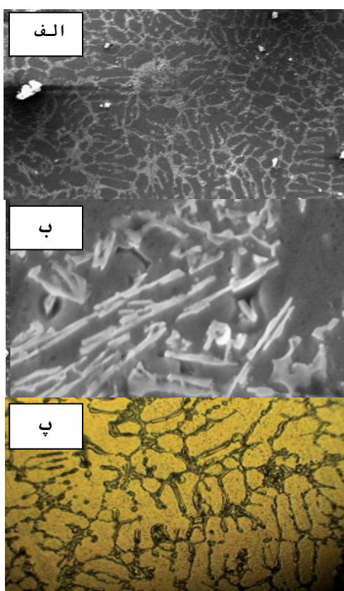
شکل (۲): ریزساختار نمونه‌های ریخته‌گری شده در دمای 750^{\circ}\text{C} با اندازه ذرات 300\text{ }\mu\text{m} : (الف) تصویر SEM با بزرگنمایی 200\times ، (ب) تصویر SEM با بزرگنمایی 2000\times و (پ) تصویر میکروسکوپ نوری با بزرگنمایی 400\times
