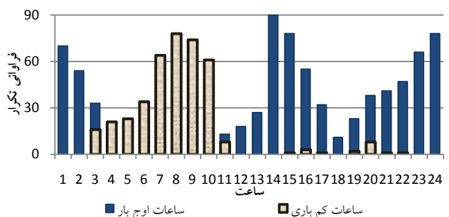
شکل ۸: فراوانی تکرار هر ساعت به عنوان ساعت TOU در فصل دوم بار
