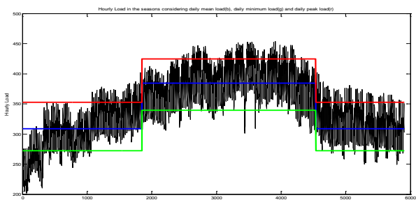
شکل ۵: بار ساعتی و مقادیر متوسط بار فصلی در استان زنجان
