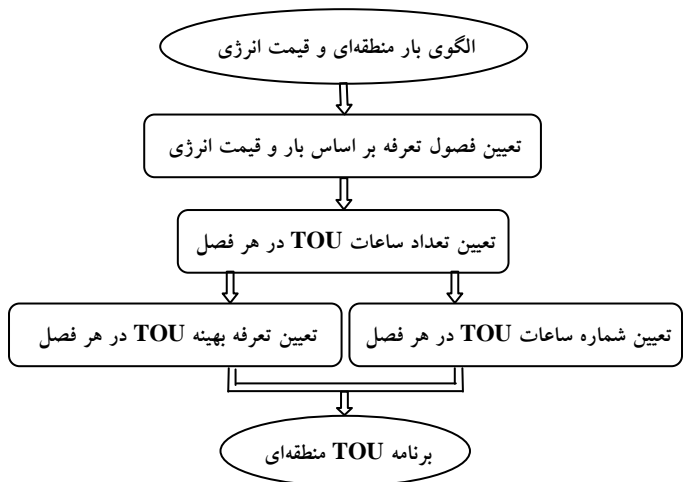
شکل ۲: فرآیند کلی طراحی برنامه TOU
