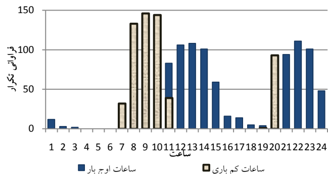
شکل ۷: فراوانی تکرار هر ساعت به عنوان ساعت TOU در فصل اول بار
