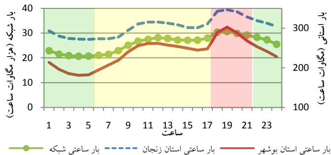
پ) بار ساعتی در تاریخ ۱۳۹۲/۹/۲
