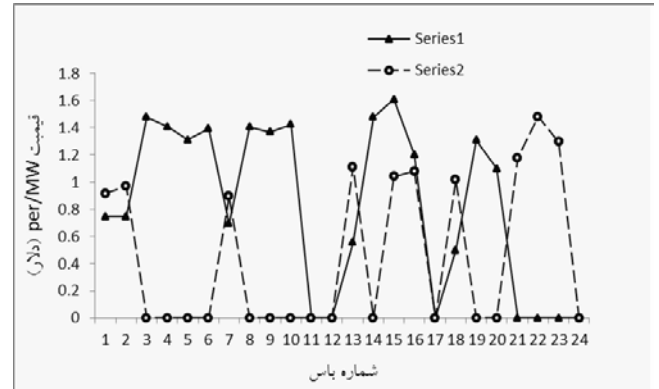
شکل (۲) نمودار قیمت باس ها در روش پیشنهادی با \alpha = 0.5
