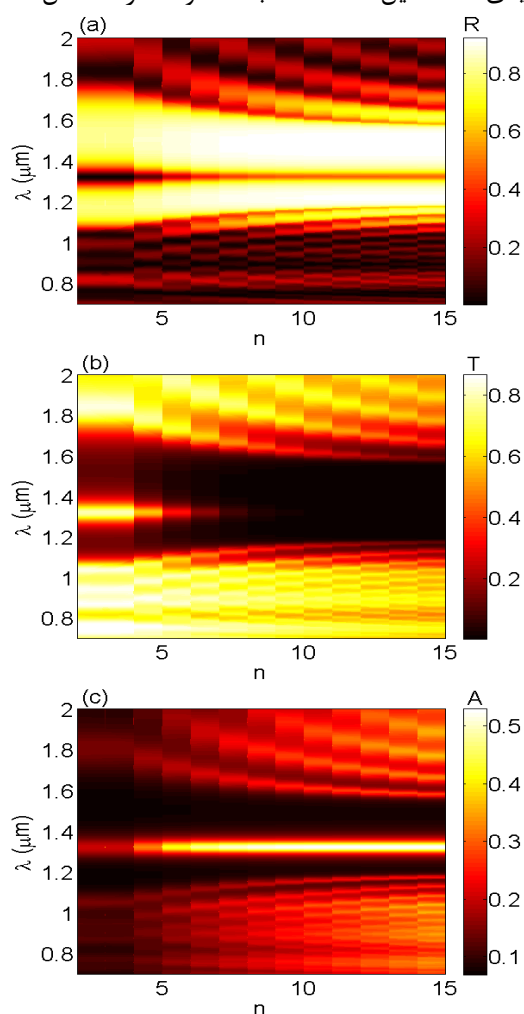
شکل ۲: طیف بازتابندگی (a)، تراگسیلندگی (b) و جذب (c) در صفحه‌ی n-\lambda برای m=3 . در اینجا \mu_c = 0.2\text{ eV} و T = 20^\circ\text{C} می‌باشد.
