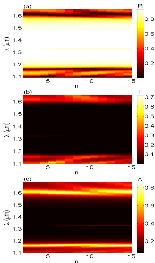
شکل ۴: طیف بازتابندگی (a)، تراگسیلندگی (b) و جذب (c) در صفحه‌ی \lambda-n برای m=10 . در اینجا \mu_c = 0.2 \text{ eV} و T = 20^{0\text{C}} می‌باشند.
