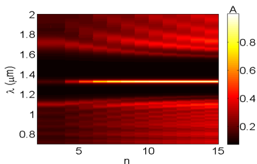
شکل ۳: طیف جذب در صفحه‌ی n-\lambda برای m=5 . در اینجا \mu_c = 0.2\text{ eV} و T = 20^\circ\text{C} می‌باشد.
