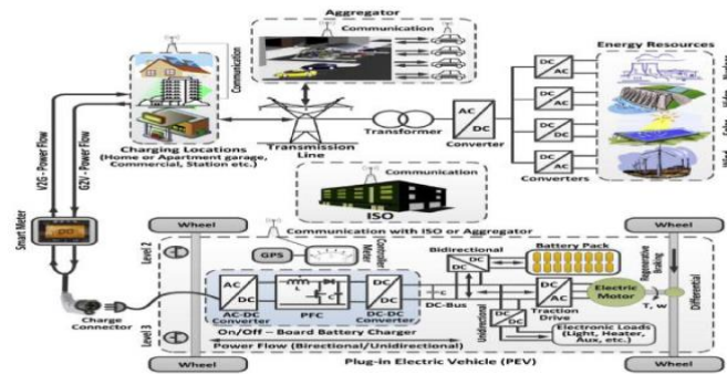
شکل ۲-۲: اجرای عمومی سیستم V2G
