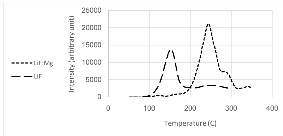
شکل (۱): مقایسه منحنی های درخشش نمونه با تابکاری و غلظت بهینه و ماده LiF خالص (منحنی LiF در عامل ۲۰ ضرب شده است)
