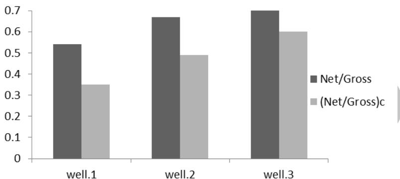
شکل 3 - مقایسه نسبت ضخامت مفید به ضخامت کل براساس مدل اشباع آب آرچی و آرچی تصحیح شده
