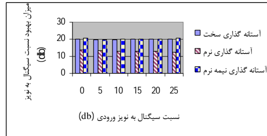
شکل (۳): ارزیابی تأثیر نوع روش آستانه‌گذاری بر میزان بهبود نسبت سیگنال به نویز ورودی در حضور نویز جمع‌شونده سفید چنانچه شکل (۳) نشان می‌دهد، ماهیت عملکردی فیلتر بانک موجک منطبق با روش آستانه‌گذاری نرم سازگاری چندانی ندارد. عملکرد فیلتر بانک برای دو نوع روش آستانه‌گذاری دیگر یکسان است.
