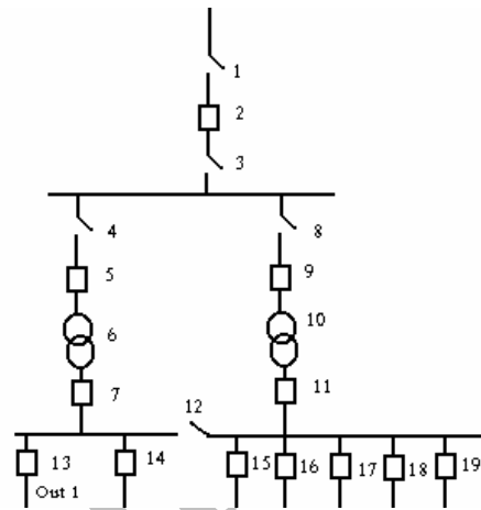
شکل (۲): دیاگرام تک خطی پست ۲۰/۶۳ kv شماره ۳ همدان
