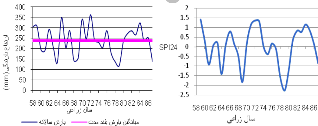
شکل ۴- تغییرات سری زمانی شاخص SPI در مقیاس زمانی ۲۴ ماهه و میزان بارندگی سالانه و متوسط بلند مدت ایستگاه اهر
