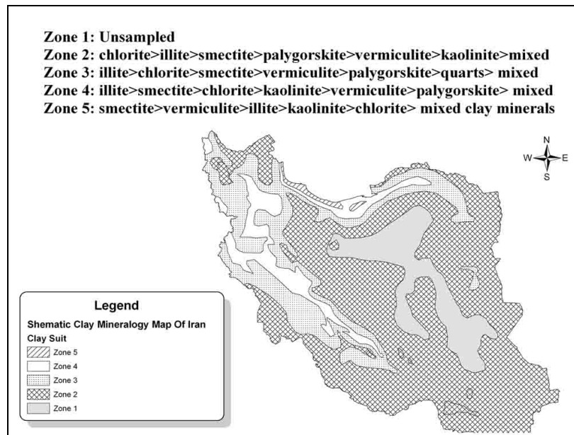
شکل ۱- نقشه شماتیک پراکنش کانیهای رس بر اساس نقشه اقلیم و نتایج به دست آمده
