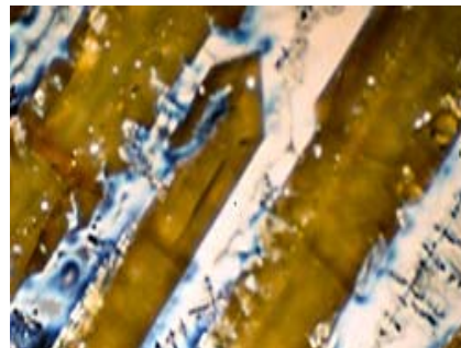
تصویر ۱. فایالیت در ماتریکس سیلیکاته با آهن بالا. بزرگنمایی \times 40
