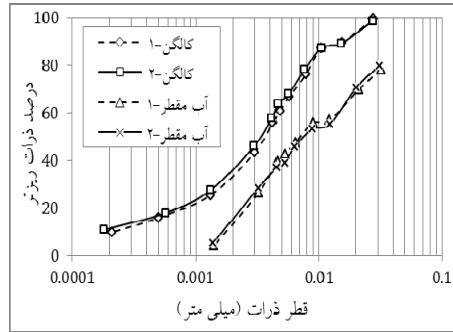
شکل ۱- منحنی دانه‌بندی
