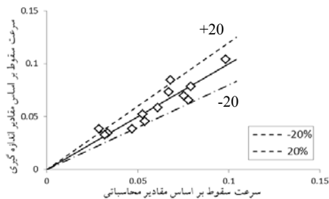
شکل ۷- مقایسه بین مقادیر مشاهده‌شده و محاسباتی برای سرعت سقوط توده‌های رسوبی
