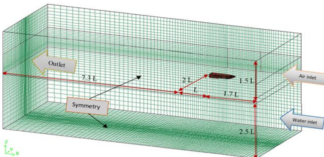
شکل (۵): ایجاد دامنه محاسباتی برای حل جریان روی شناور.
