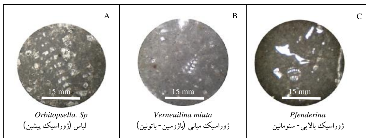
شکل 2. تعیین سن میکروفسیل‌های فرامینفرهای بتتیک؛ نمونه گرفته شده از بلوک‌های آهکی دولومیتی شده از سری تاشک؛ منطقه ریحان.
