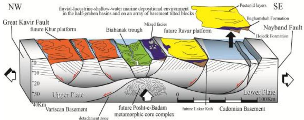
شکل 4. مدل ارائه شده برای ریفت بلوک طبس.
