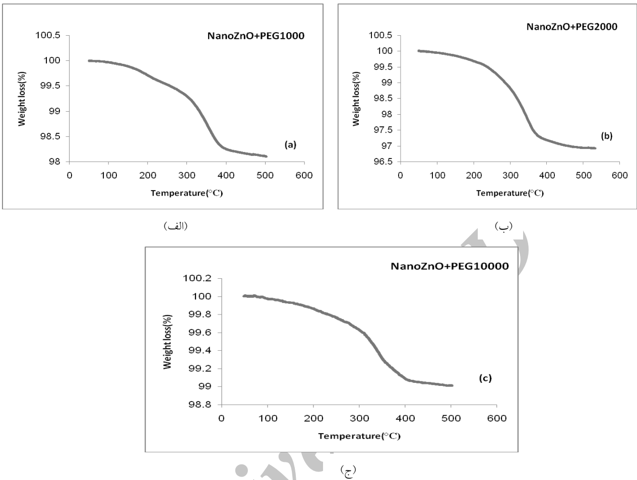
شکل (۶) نمودارهای گرما وزن سنجی از نمونه های (الف) NanoZnO+PEG1000، (ب) NanoZnO+PEG2000 و (ج) NanoZnO+PEG10000
