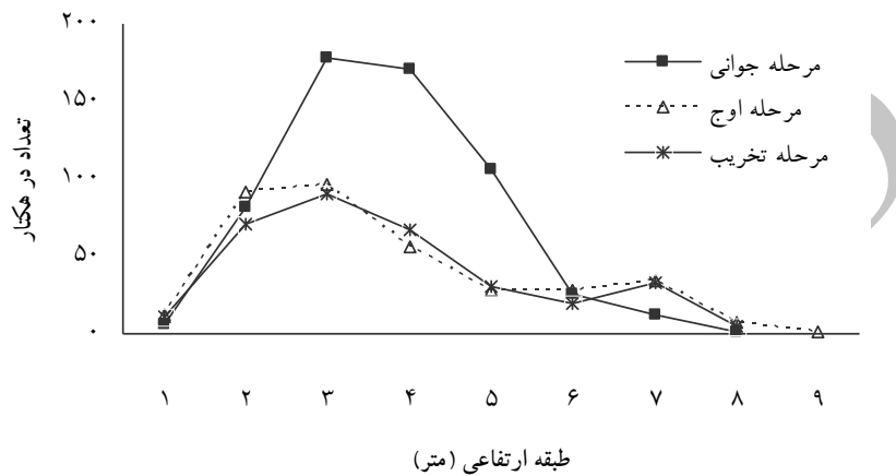
شکل ۲- توزیع تعداد در طبقه‌های ارتفاعی در مراحل مختلف تحولی راش-ممرز در طرح حاجی کلا- تیرانکلی
