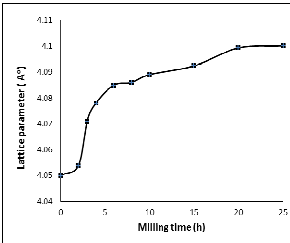
شکل ۸: تغییرات پارامتر شبکه آلومینیوم بر حسب زمان آسیاب کاری در آلیاژ آلومینیوم ۷.۵
