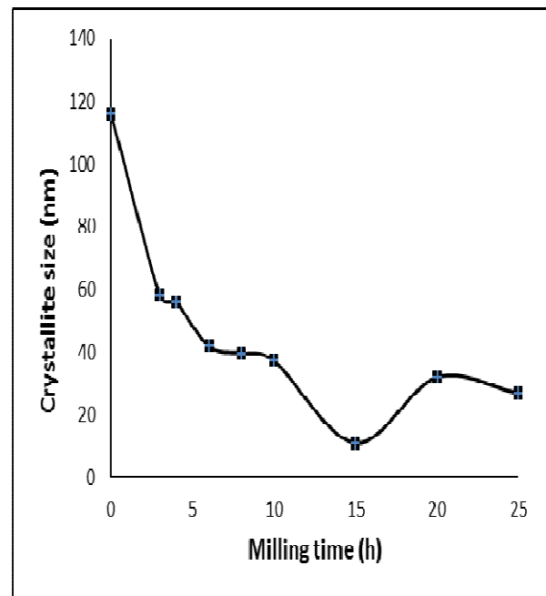
شکل ۶: تغییرات اندازه بلورک های آلومینیوم ۷.۵ بر حسب زمان آسیاب کاری
