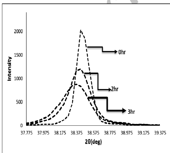
شکل ۲: جابجایی پیک (۱۱۱) آلومینیوم بر حسب زمان آسیاب کاری
