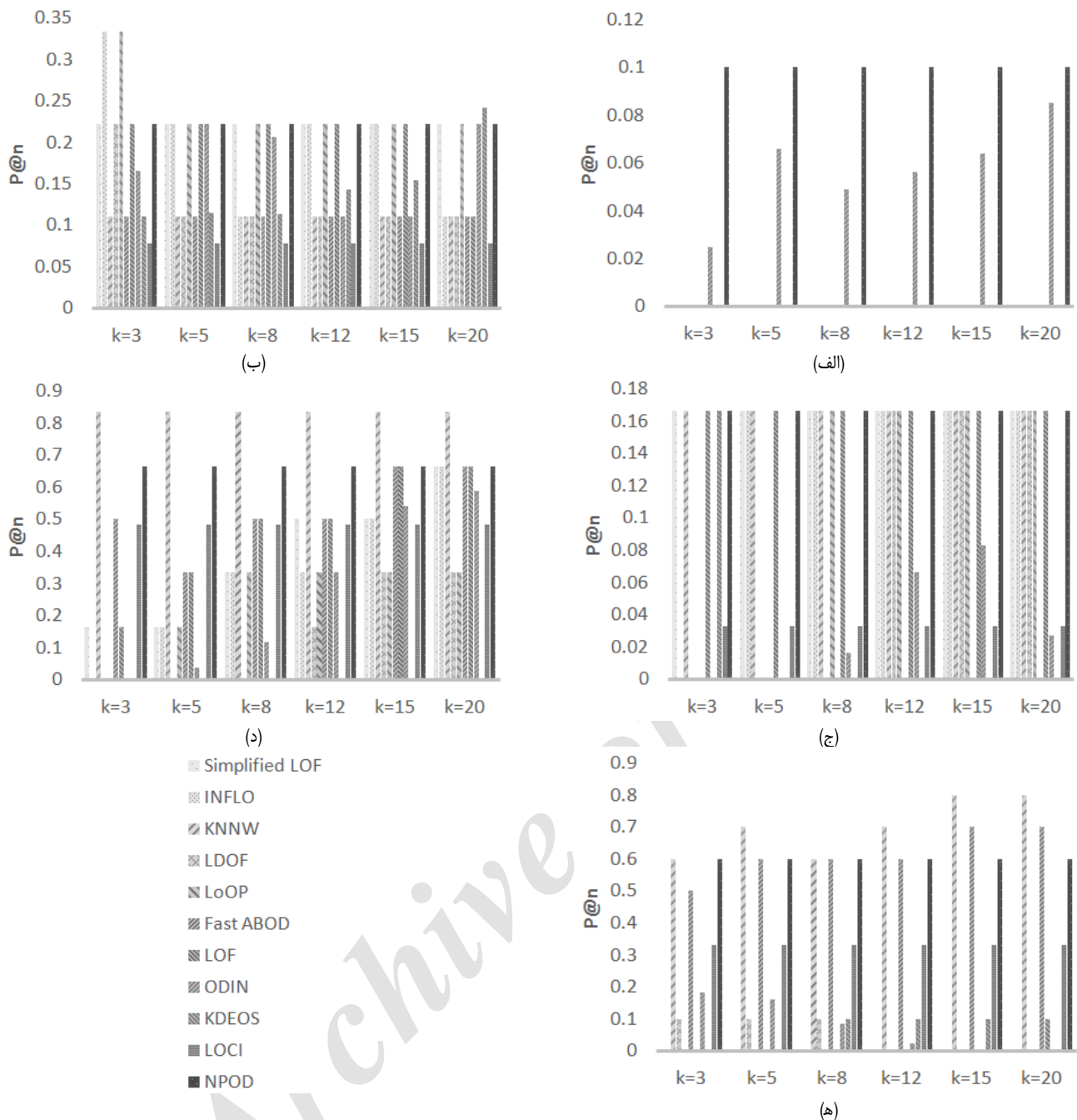
شکل ۵: ارزیابی نتایج آزمایش‌های با معیار \text{precision at } n بر روی مجموعه داده‌های (الف) Pima، (ب) Glass، (ج) Stamps، (د) Lymphography و (ه) WBC.
