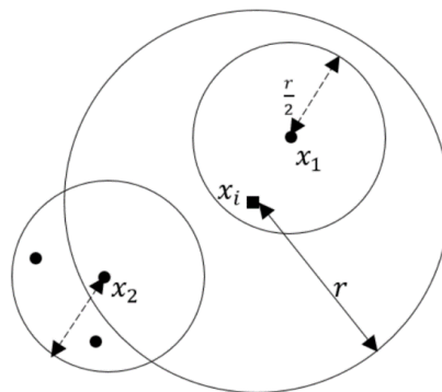
شکل ۱: نمایش شعاع r -همسایگی نقطه x_i شامل همسایگان x_1 و x_2 و شعاع r/2 همسایگی برای هر یک از همسایگان x_i .
