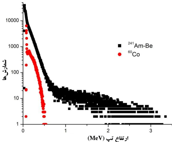
شکل ۵. طیف‌های انرژی به دست آمده برای تابش چشمه Am-Be و چشمه ^{60}\text{Co} .
