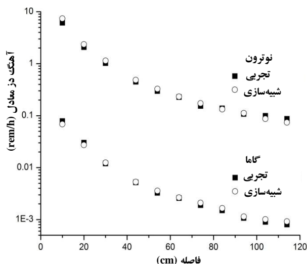
شکل ۶. تغییرات آهنگ دز معادل با فاصله‌ی دزیتر از چشمه.
