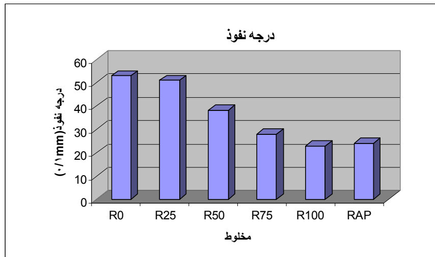
شکل ۴. نمودار مقایسه‌ای درجه نفوذ قیر ترکیبی برای مخلوط‌های مختلف
