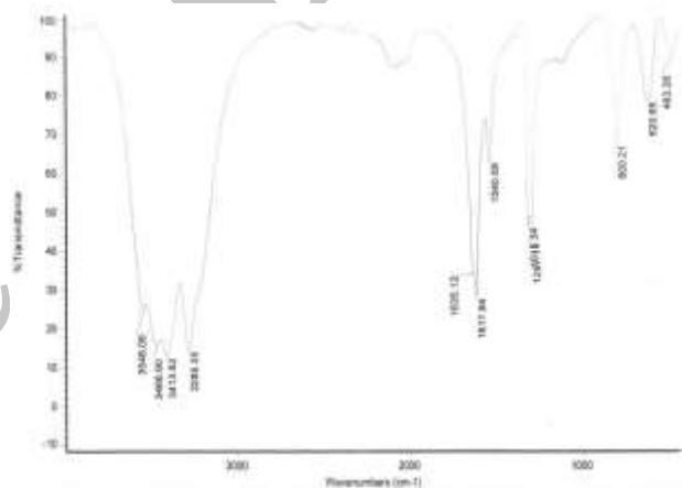
شکل ۲: طرح شماتیک حاصل از آنالیز FTIR مربوط به سیس پلاتین اولیه
