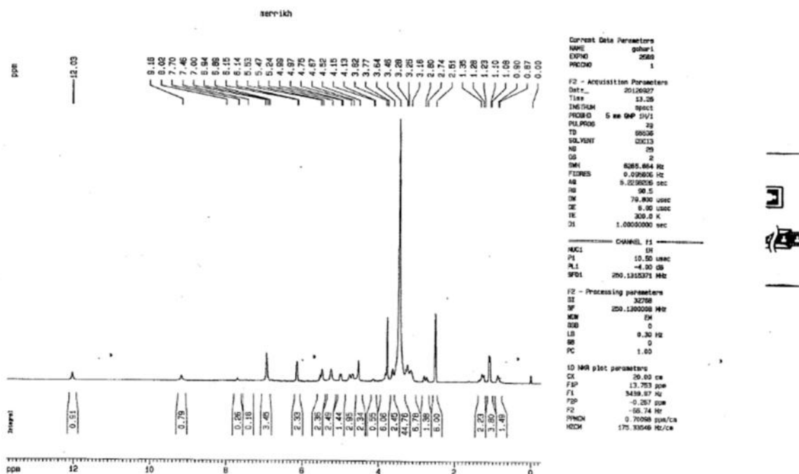
شکل ۱- طیف 1 H-NMR
