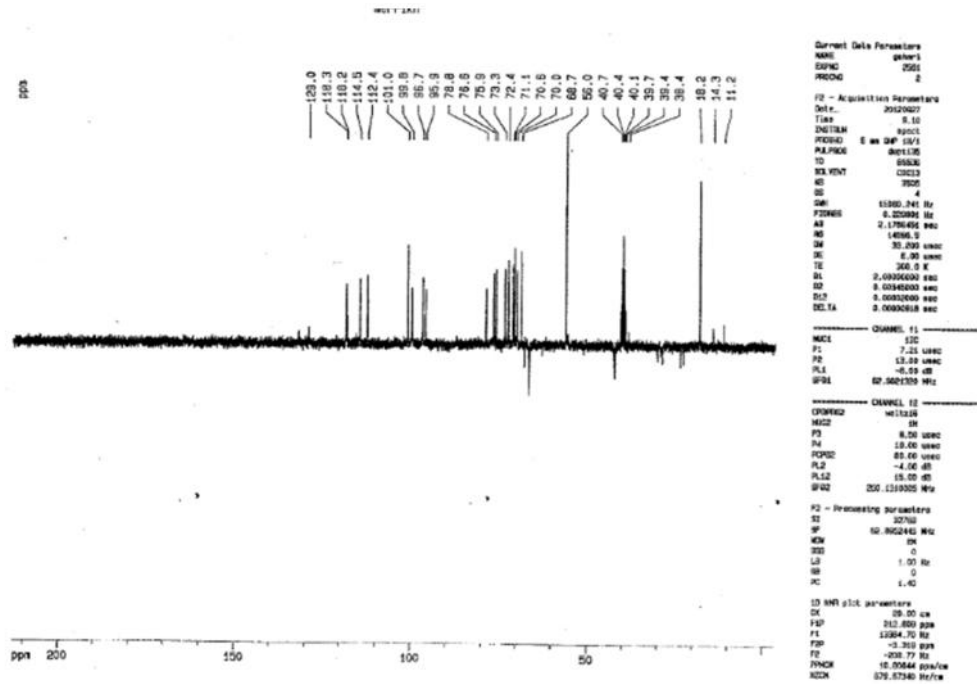
شکل ۳- طیف 135 dept
