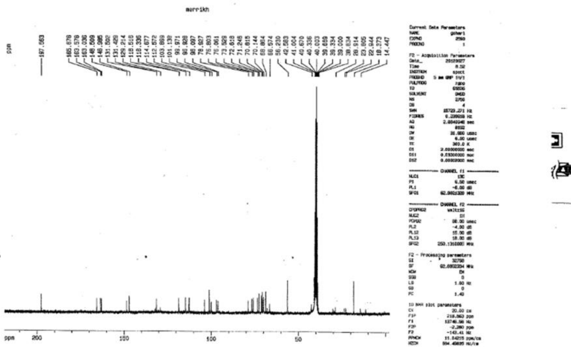
شکل ۲- طیف 13 C-NMR
