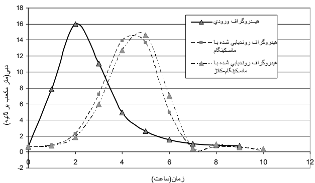
شکل ۷. روندیابی سیل ۵ ساله با روش ماسکینگام و ماسکینگام-کانز
