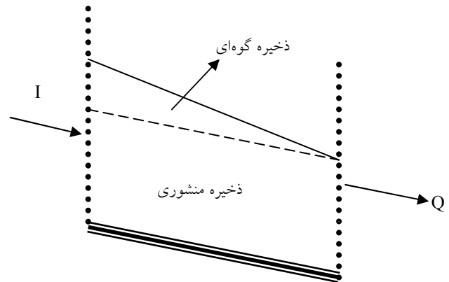
شکل ۲. انواع ذخیره در موقع حرکت موج سیل
