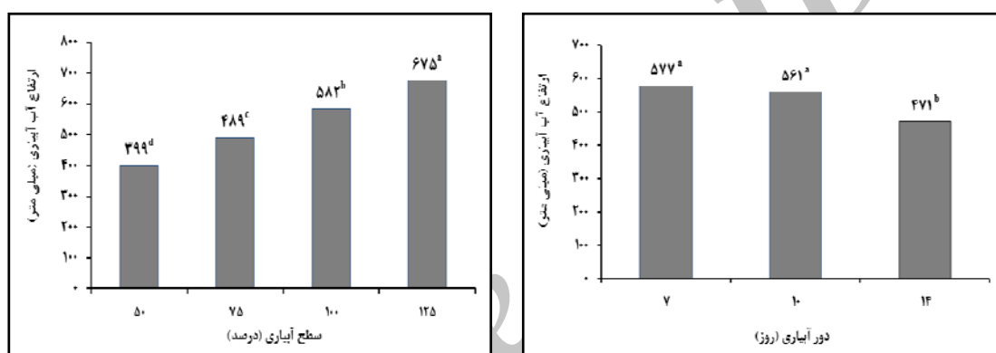
شکل ۳- مقایسه میانگین میزان آب مصرف شده در تیمارهای مختلف دور و سطح آبیاری
