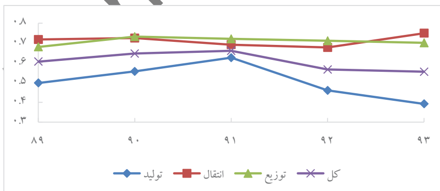
نمودار ۱. میانگین نمرات کارایی کل شبکه برق و بخش‌های تشکیل دهنده‌ی آن در بازه زمانی ۱۳۸۹-۱۳۹۳
