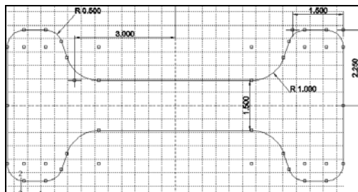
شکل ۲: شکل و ابعاد قالب تمام‌کننده.
