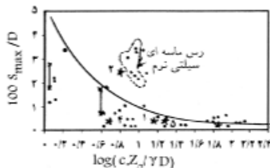
شکل ۷- ارتباط مقادیر نشست نسبی ( S_{max} / D ) با نسبت ( cz_0 / \gamma D ) (شماره‌ها، شماره ردیف تونلها در جدول شماره ۱ می‌باشد)
