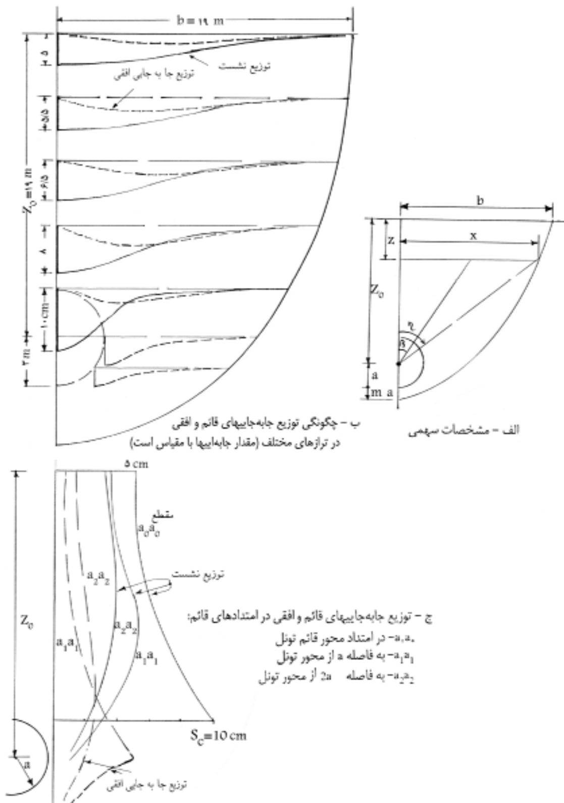
شکل ۸- الگوی جابه‌جاییهای قائم و افقی اطراف و بالای تونل (نصف مقطع) بر اساس رابطه‌های ۵ و ۱۳
