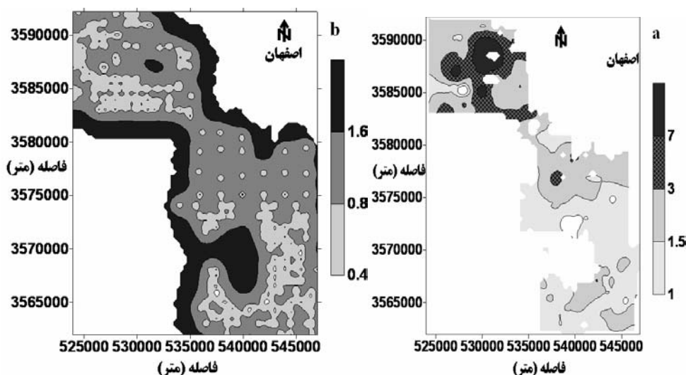
شکل ۴- کریجینگ قطعه‌ای (a) و واریانس تخمین (b) سرب قابل جذب در خاک (میلی‌گرم بر کیلوگرم).
