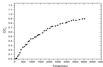
شکل شماره ۶): منحنی شکست ستون بستر ثابت کربن فعال در حذف رنگ AB1
