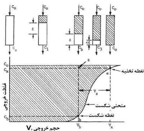
شکل شماره (۴): منحنی ایده آل شکست ستون
