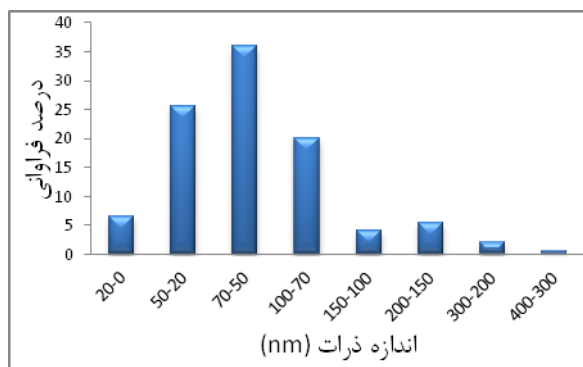
شکل ۱۰. توزیع اندازه ذرات نمونه ۴.
