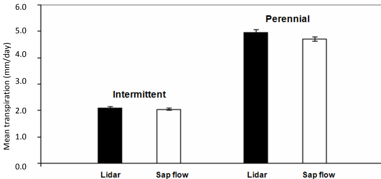
(شکل ۷) - برآورد میانگین روزانه تعرق از لایدار در مقابل مقدار میانگین روزانه تعرق اندازه گیری شده از گردش عصاره ای درخت برای سایت‌های
