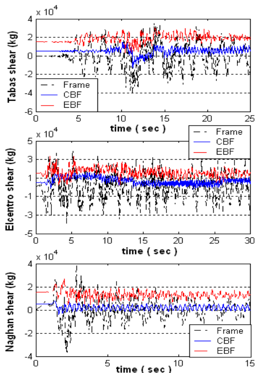
شکل (۱۱). تاریخچه زمانی برش در پای ستون‌های طبقه اول، قاب ۵ طبقه و ۲ دهانه با اتصال نبشی
