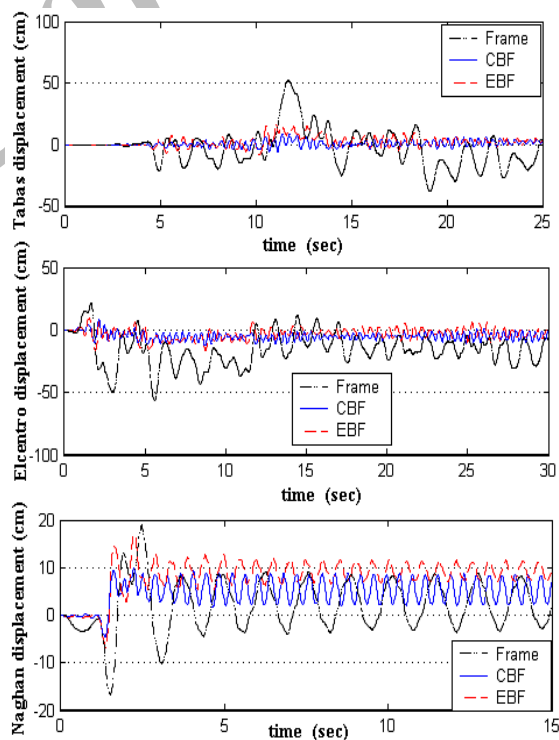
شکل (۹). تاریخچه تغییر مکانی گره بام در قاب ۵ طبقه و ۴ دهانه با اتصال نبشی
