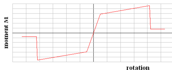
شکل (۱). منحنی لنگر - دوران اتصال نیمه صلب
