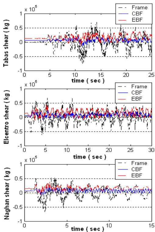
شکل (۱۳). تاریخچه زمانی برش در پای ستون‌های طبقه اول، قاب ۱۰ طبقه و ۲ دهانه با اتصال نبشی
