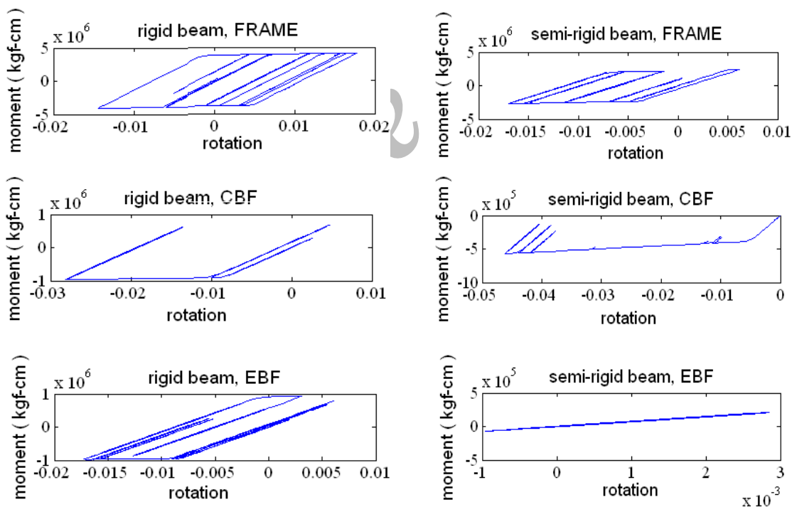
شکل (۲۰). قاب ۱۰ طبقه و ۳ دهانه با اتصال سپری
