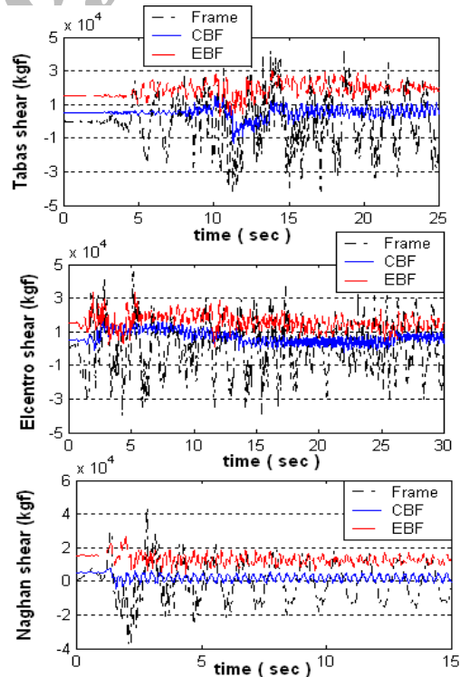
شکل (۱۲). تاریخچه زمانی برش در پای ستون‌های طبقه اول، قاب ۵ طبقه و ۲ دهانه با اتصال سپری
