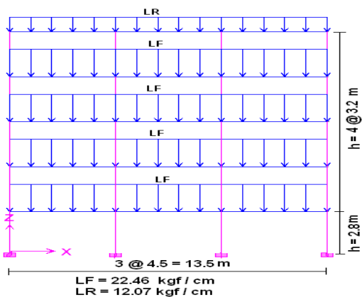
شکل (۳). نمای کلی از قاب ۵ طبقه، ۳ دهانه
