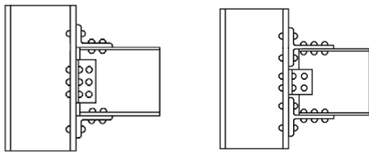
شکل (۵). هندسه اتصالات نیمه صلب
