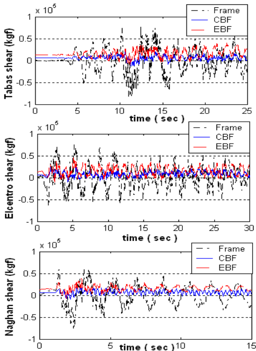
شکل (۱۴). تاریخچه زمانی برش در پای ستون‌های طبقه اول، قاب ۱۰ طبقه و ۲ دهانه با اتصال سپری
