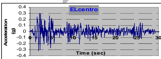
شکل (۶). شتاب‌نگاشت‌های مقیاس شده به g
