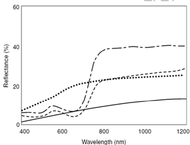
شکل ۱: طیف انعکاسی اجزاء طبیعی: — برگ درخت لیمو، ..... خشک، - - - برگ درخت صنوبر، — خاک [۵].
