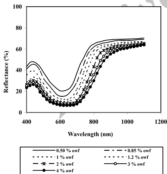
شکل ۶: منحنی انعکاس پارچه‌های رنگزای شده با رنگزای Vat Blue 6 در غلظت‌های مختلف رنگزای.
