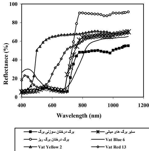
شکل ۵: منحنی انعکاس پارچه‌های رنگزای شده با مواد رنگزای خمی (به صورت تکرنگ) با غلظت رنگزای (owf) ۲٪ در کنار منحنی انعکاس برگ سبز.
