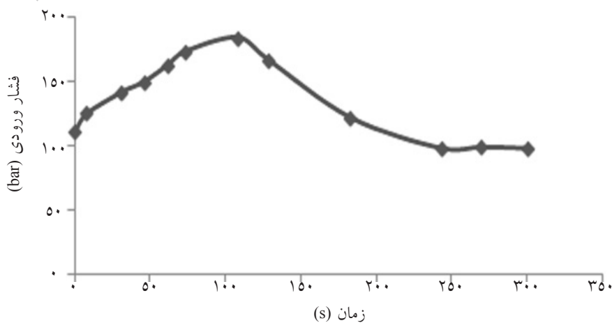
شکل ۹- تغییرات فشار ورودی در سرعت تزریق 0.5 cc/min
