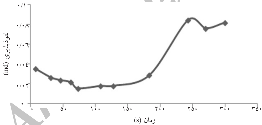
شکل ۸- تغییرات نفوذپذیری در زمان‌های اولیه تزریق با نرخ 0.5 cc/min
