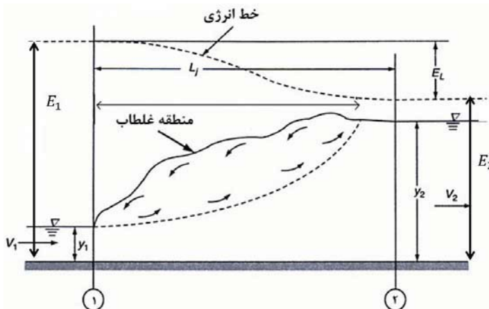
شکل ۱- جهش آبی بر روی بستر صاف
