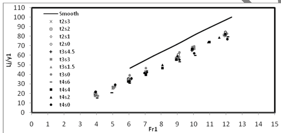
شکل ۷- تغییرات طول نسبی جهش آبی با عدد فرود در بستر صاف و بسترهای زیر برای کلیه آزمایشها
