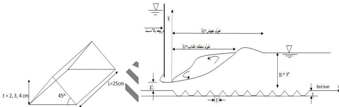
شکل ۳- طرح شماتیک جهش آبی بر روی بستر زبر
