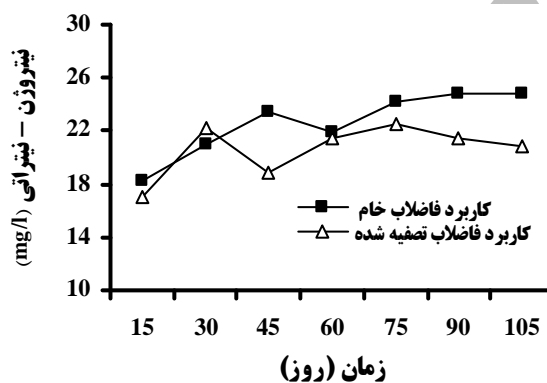
(شکل ۵) - تغییرات میانگین مقدار نیتروژن-نیتراتی در زه‌آب خروجی از ستون‌های خاک در طول زمان
