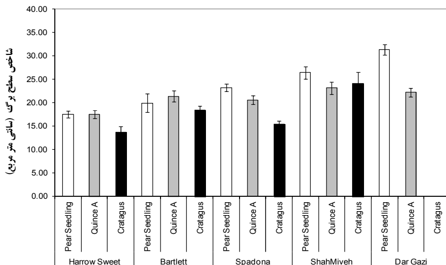
شکل ۸- متوسط میزان شاخس سطح برگ در برگ‌های در ارقام گلابی روی سه پایه مختلف. برای رقم درگزی روی پایه زالک به دلیل عدم سازگاری فاقد داده است.
