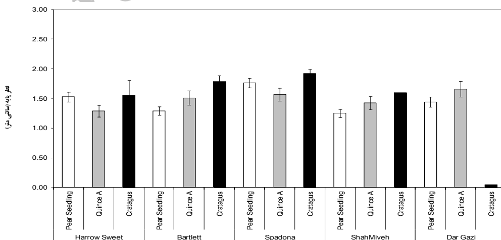
شکل ۲- قطر پایه در نهال ارقام گلابی روی سه پایه مختلف گلابی، به و زالک.
