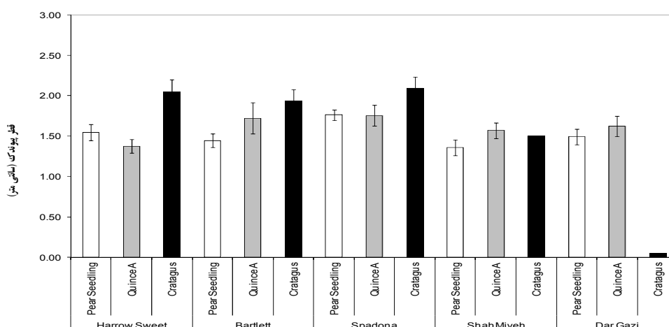
شکل ۳- قطر پیوندک در نهال ارقام گلابی روی سه پایه مختلف گلابی، به و زالک. رقم درگزی روی پایه زالک به دلیل عدم سازگاری فاقد داده است
