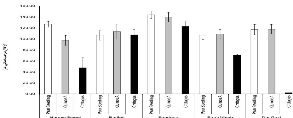
شکل ۴- ارتفاع درخت در ارقام گلابی روی سه پایه مختلف گلابی، به و زالک. رقم درگزی روی پایه زالک به دلیل عدم سازگاری فاقد داده است.
