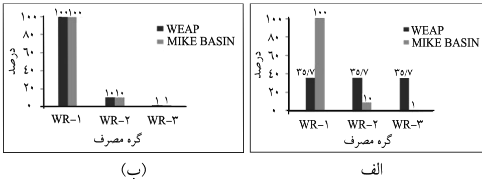
شکل ۲- نتایج به‌دست آمده از اجرا دو مدل در شرایط الف) اولویت یکسان گره‌های مصرف و ب) اولویت متفاوت.
