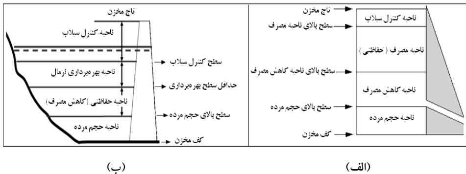
شکل ۶- نواحی بهره‌برداری در مخازن (الف) WEAP و (ب) MIKE BASIN
