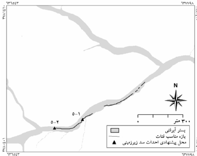
شکل ۱۰- نقشه محل‌های پیشنهادی احداث سد زیرزمینی بر روی قنات دهن چنار.
