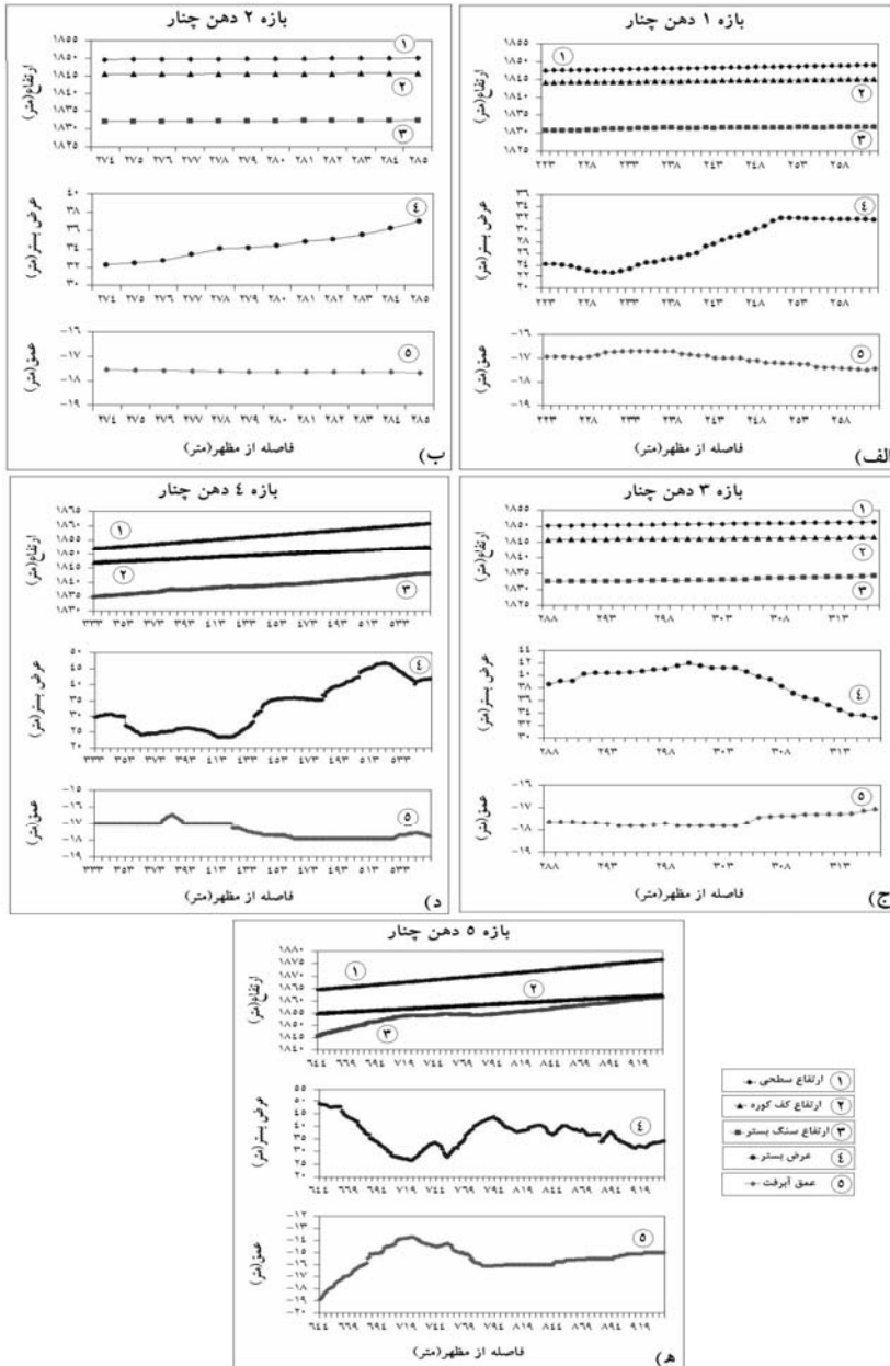
شکل ۸- تغییرات ارتفاع سطح بستر، ارتفاع کف کوره، ارتفاع سنگ بستر، عرض بستر و عمق آبرفت در طول بازه‌های قنات دهن چنار.
