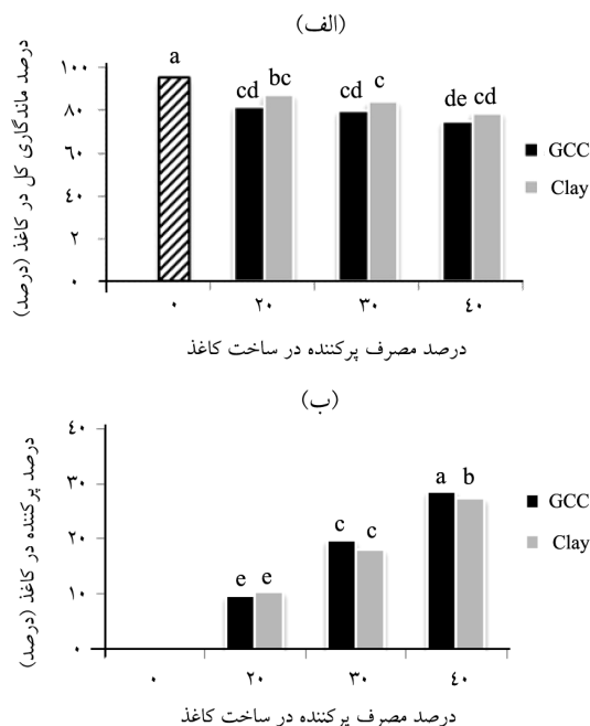
شکل ۱- رابطه درصد مصرف پرکننده در ساخت کاغذ با درصد ماندگاری کل (الف) درصد پرکننده باقی مانده در کاغذ (ب).
