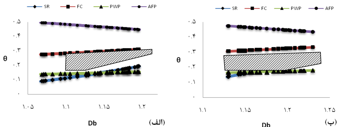
شکل ۱- تغییرات ثابت‌های رطوبتی LLWR با وزن مخصوص ظاهری الف) خاکورزی مرسوم ب) بدون خاکورزی
