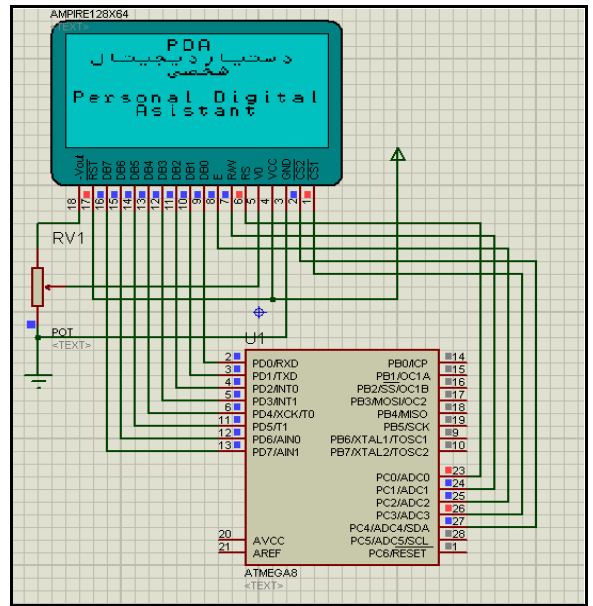
شکل ۱: مدل شبیه سازی شده سیستم PDA
