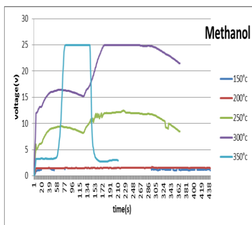
شکل (۱۰): واکنش نانو حساسه به تغییرات دمایی در غلظت 200ppm متانل
