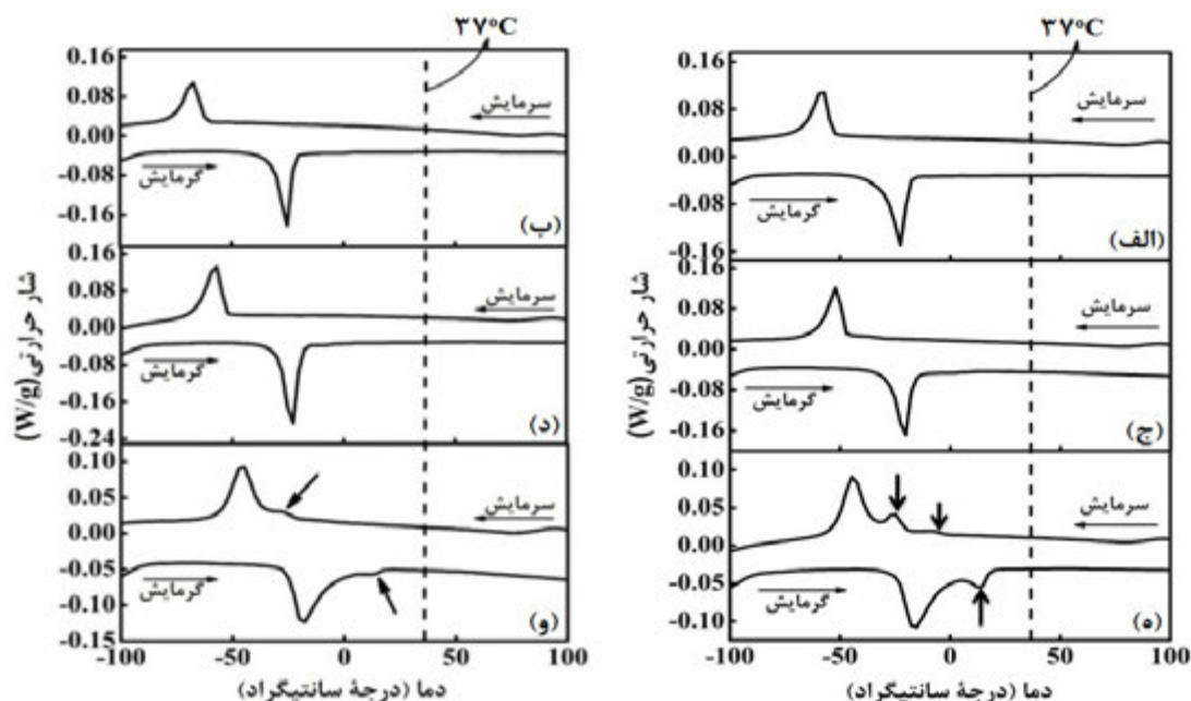
شکل (۵): منحنی‌های DSC نمونه‌های (الف): ۴۰ و (ب): ۶۰ درصد کارسرد شده و به مدت ۱۰ دقیقه در دمای ۶۰۰°C عملیات حرارتی آنیل شده، (ج): ۴۰ و (د): ۶۰ درصد کارسرد شده و به مدت ۳۰ دقیقه در دمای ۶۰۰°C عملیات حرارتی آنیل شده و (ه): ۴۰ و (و): ۶۰ درصد کارسرد شده و به مدت ۹۰ دقیقه در دمای ۶۰۰°C عملیات حرارتی آنیل شده
